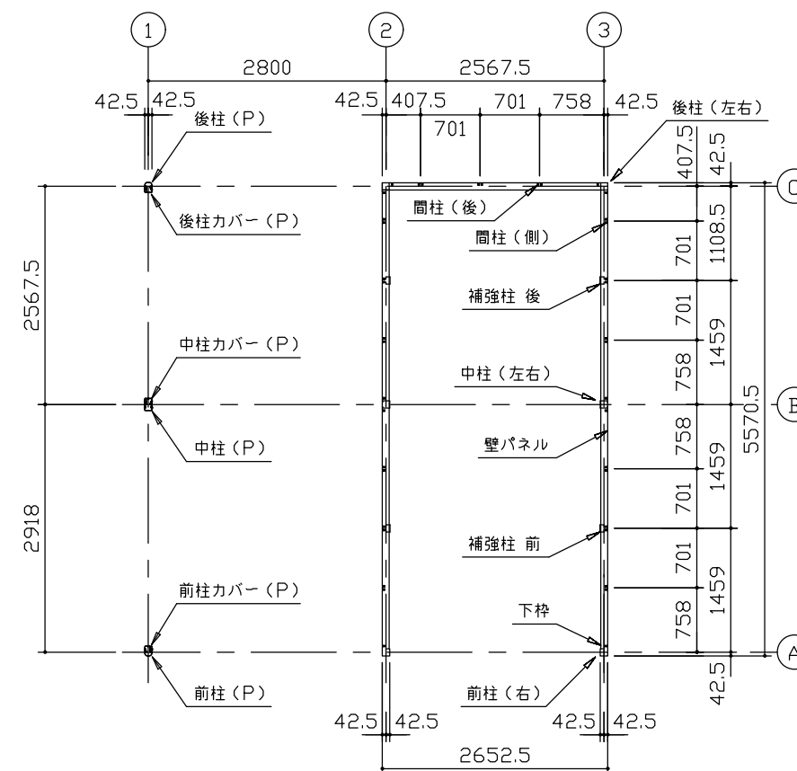
平面図 (S=1/80)
