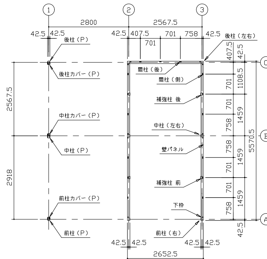
平面図 (S=1/80)
