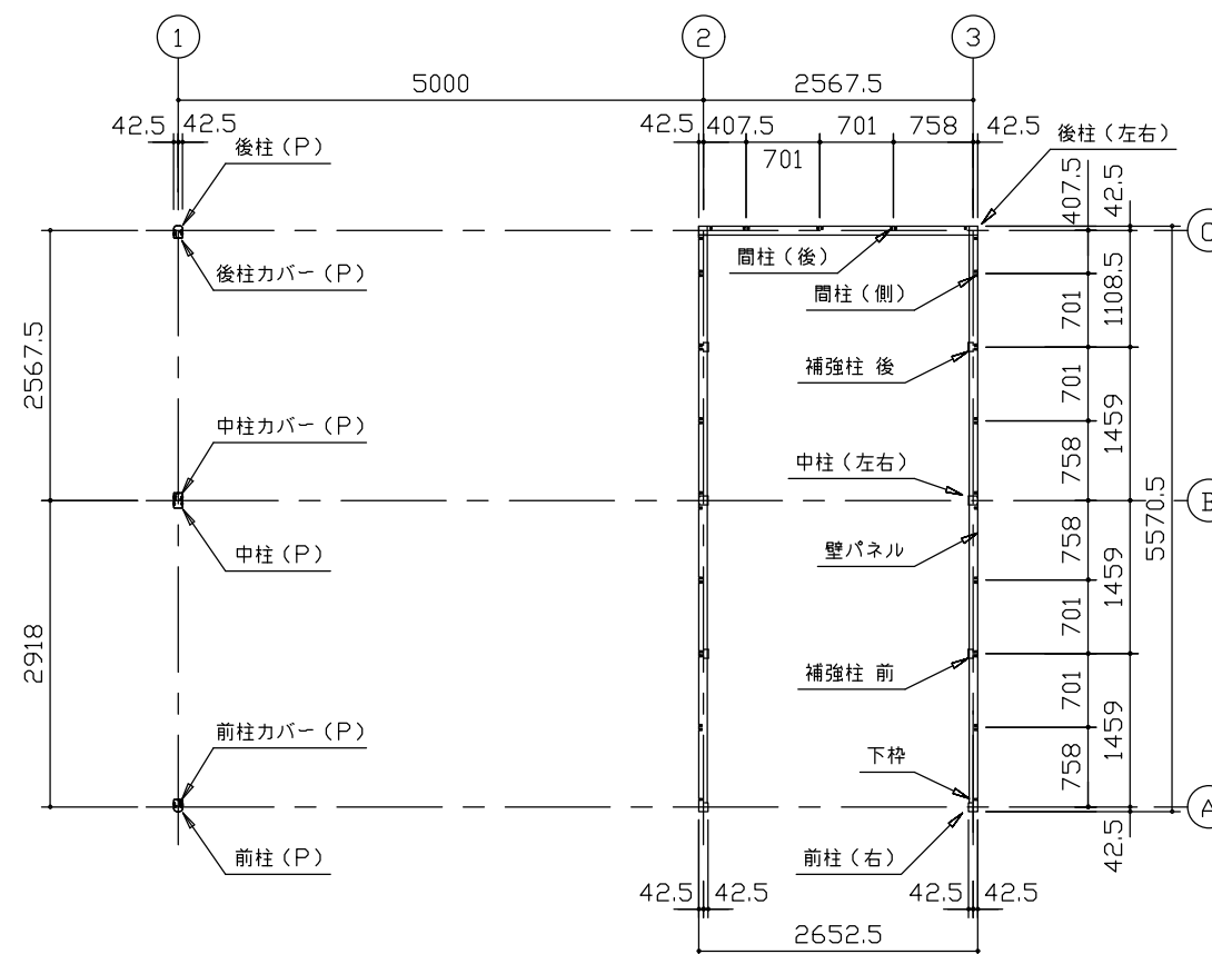
平面図 (S=1/80)
