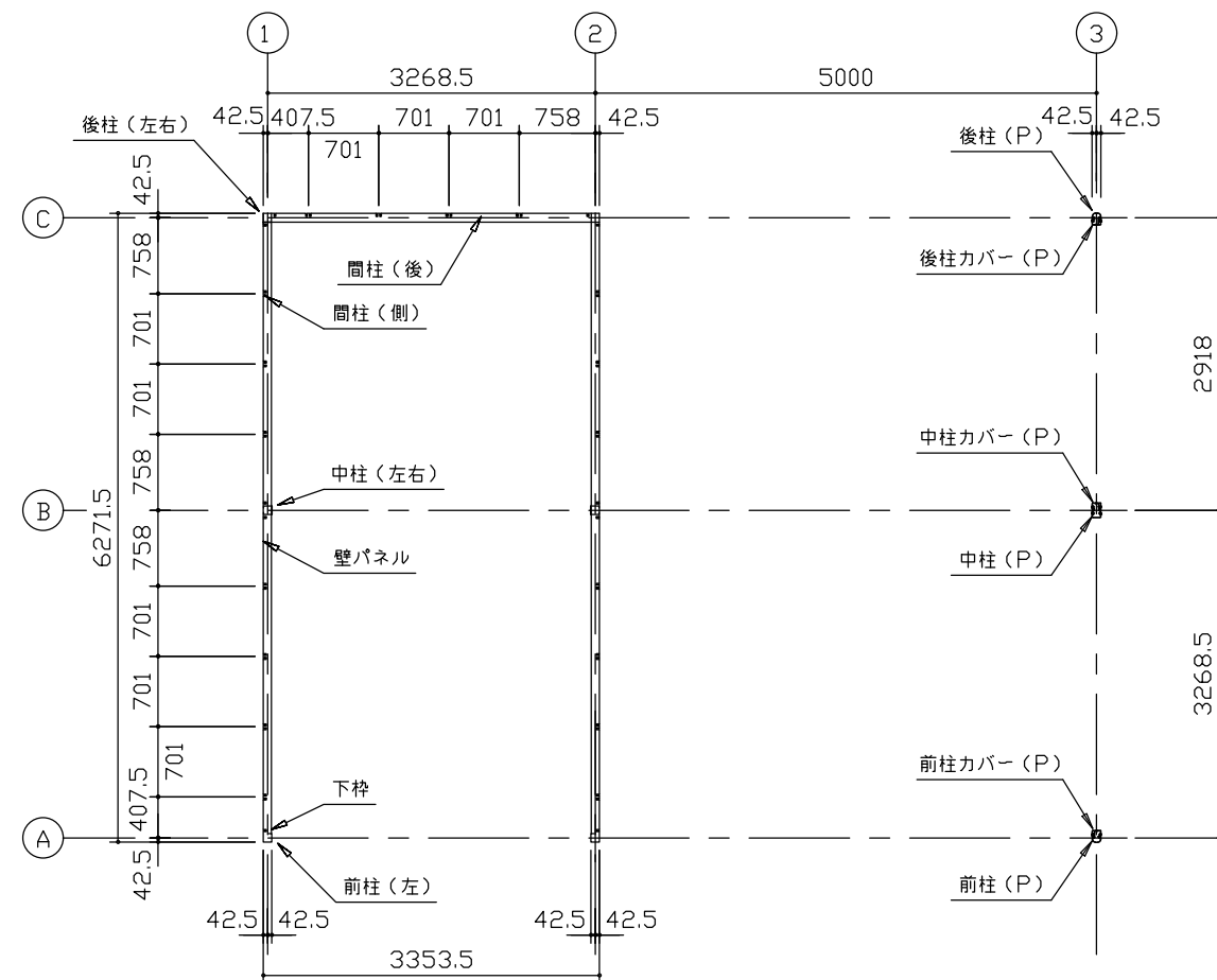
平面図 (S=1/80)
