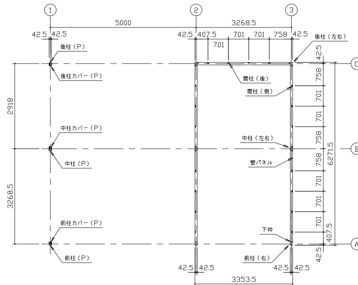
平面図 (S=1/80)
