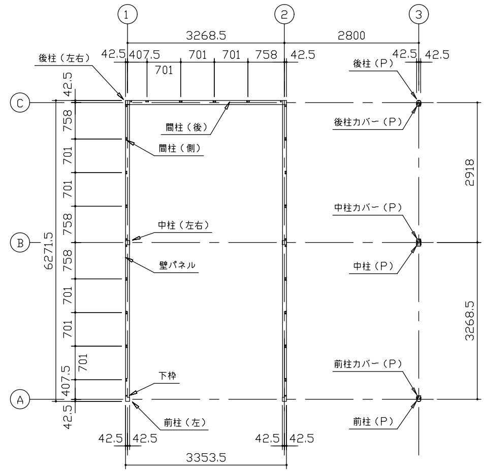
平面図 (S=1/80)
