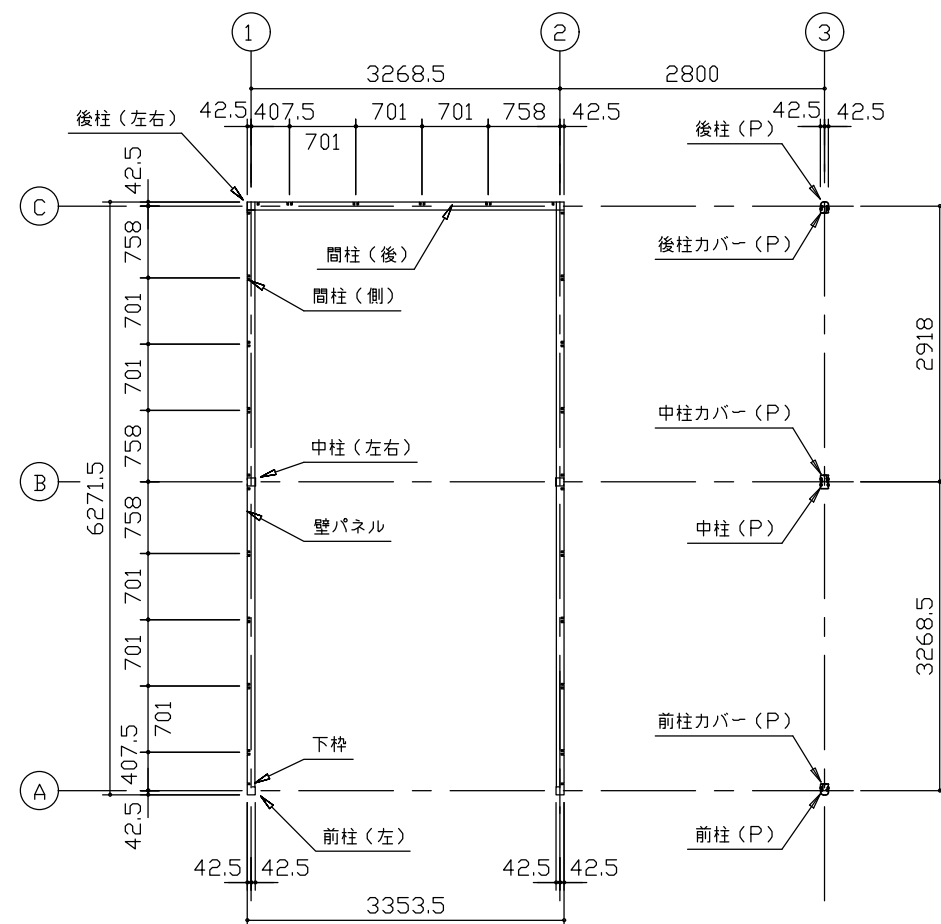
平面図 (S=1/80)
