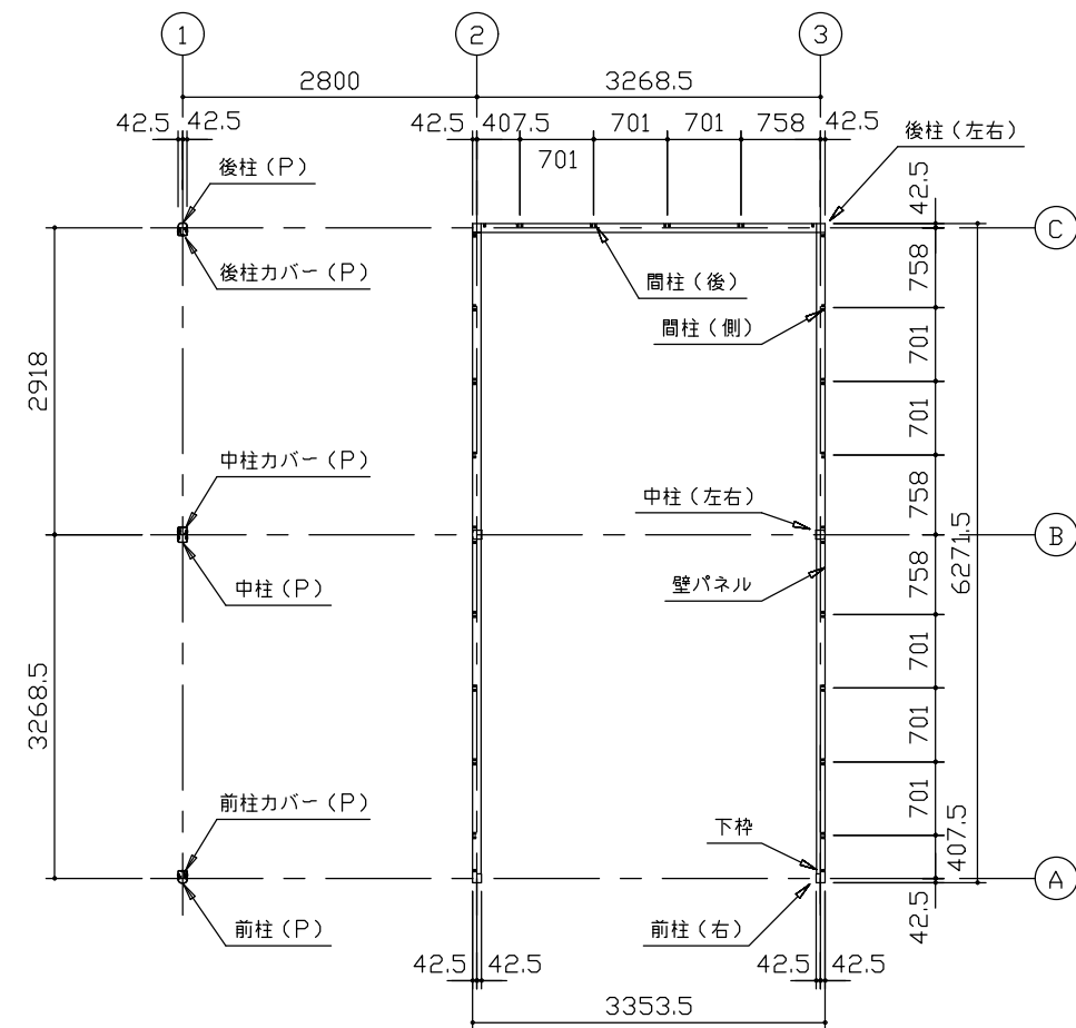
平面図 (S=1/80)
