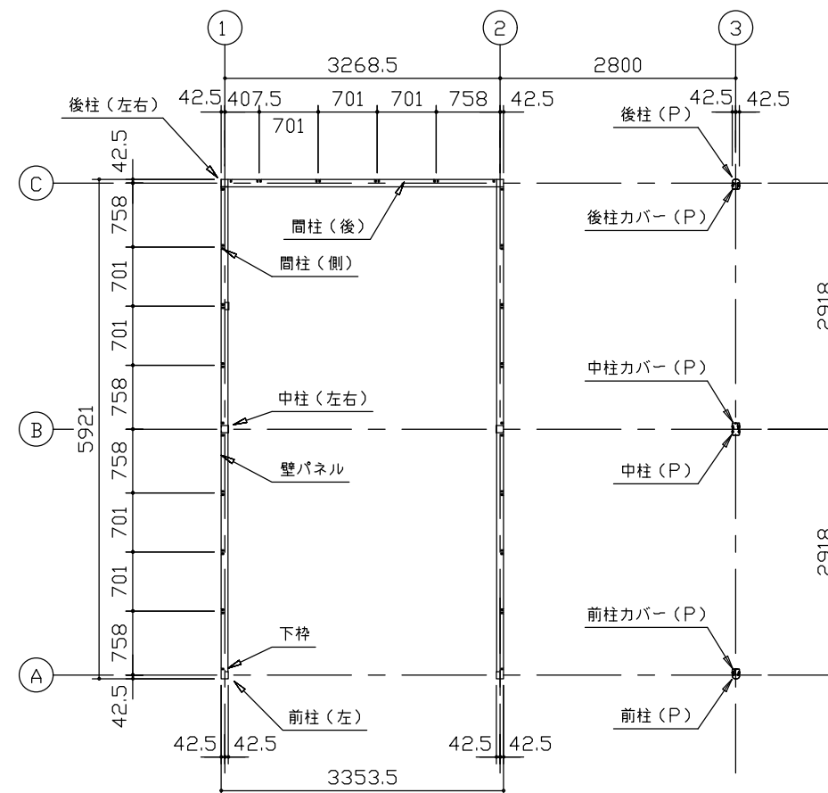
平面図 (S=1/80)
