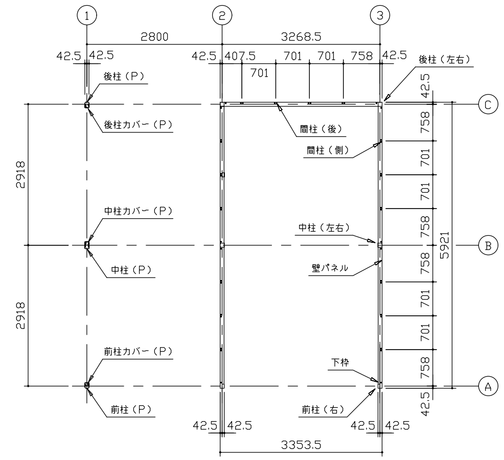
平面図 (S=1/80)
