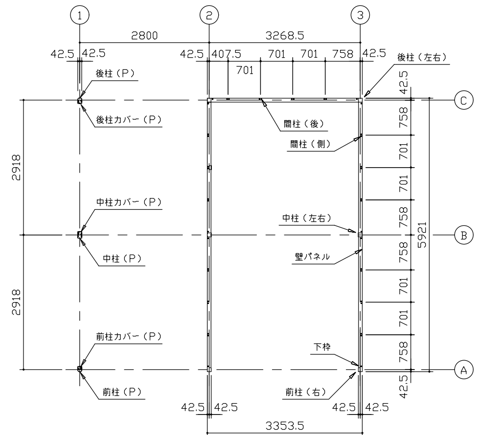
平面図 (S=1/80)
