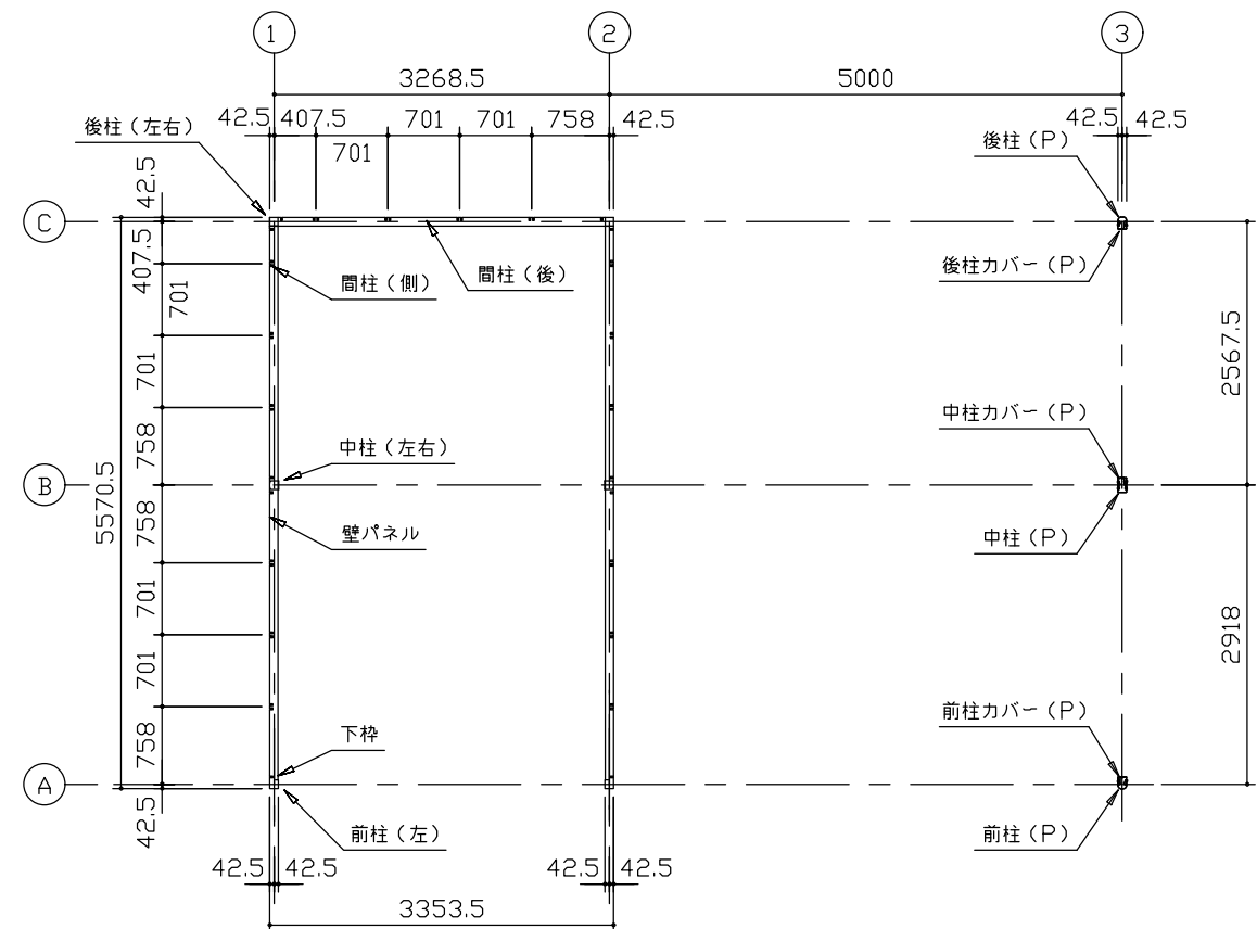
平面図 (S=1/80)
