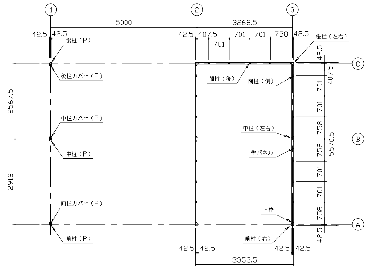
平面図 (S=1/80)
