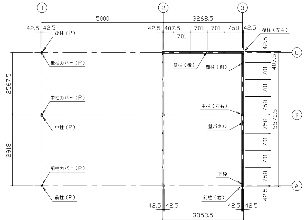
平面図 (S=1/80)
