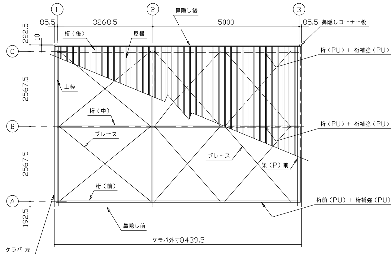
小屋伏図 (S=1/80)
