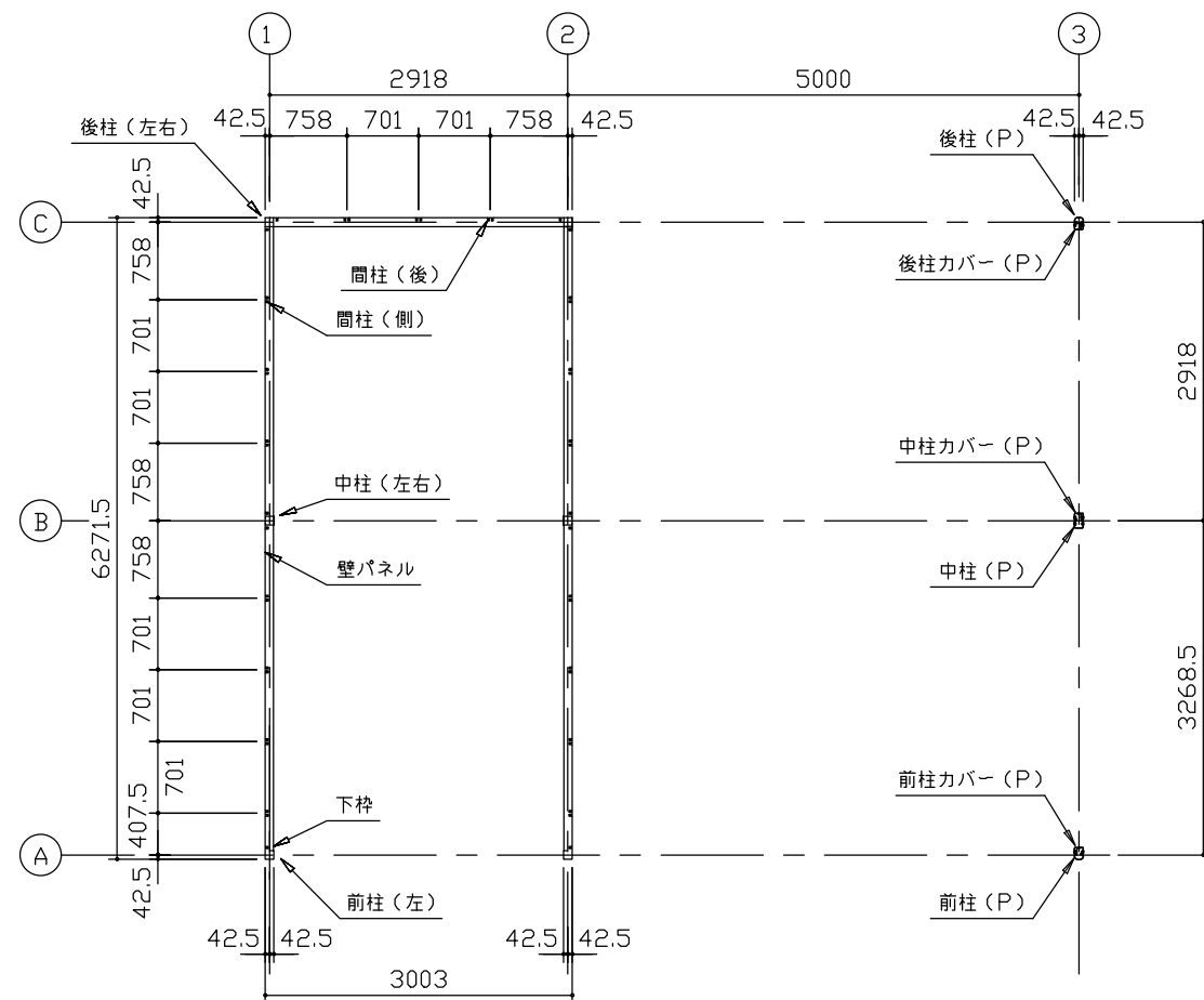
平面図 (S=1/80)
