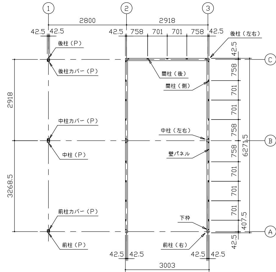
平面図 (S=1/80)
