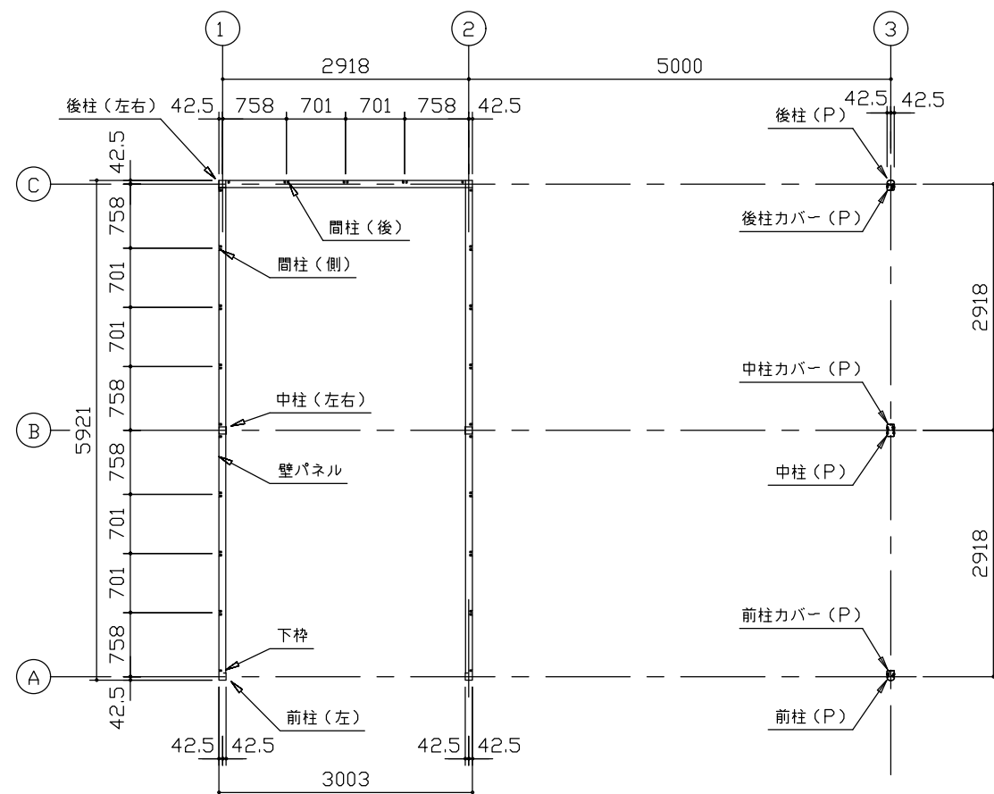
平面図 (S=1/80)
