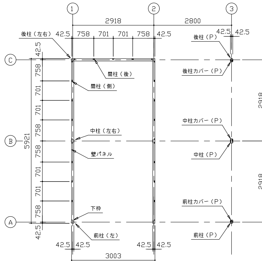
平面図 (S=1/80)
