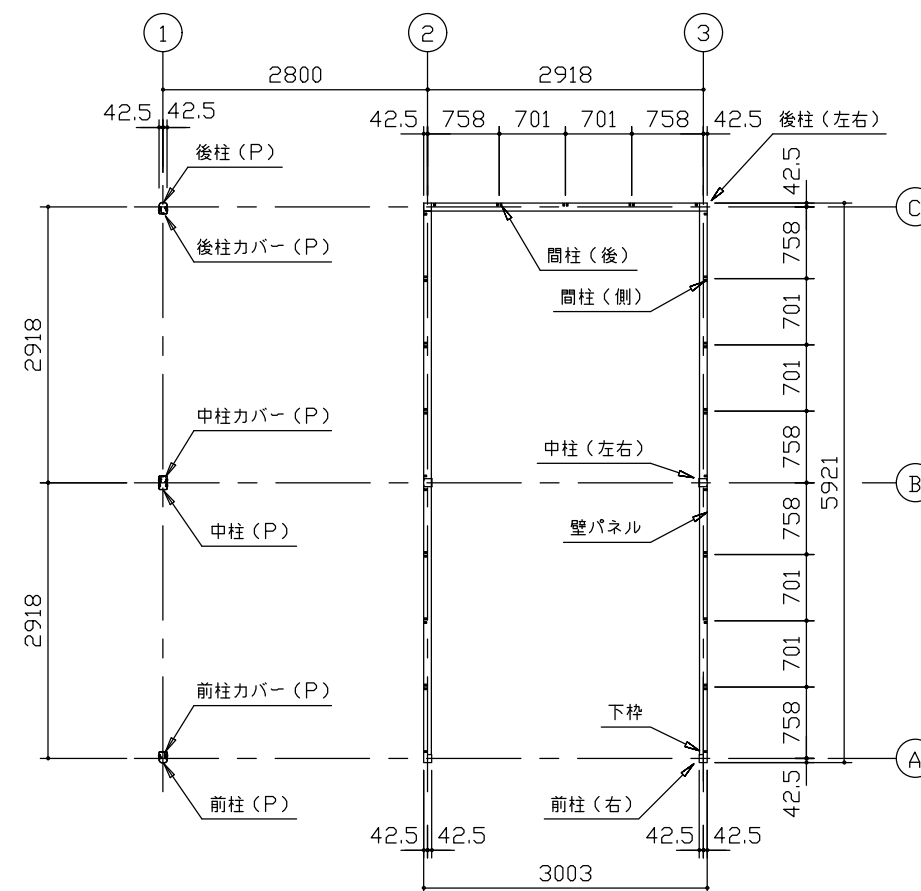
平面図 (S=1/80)
