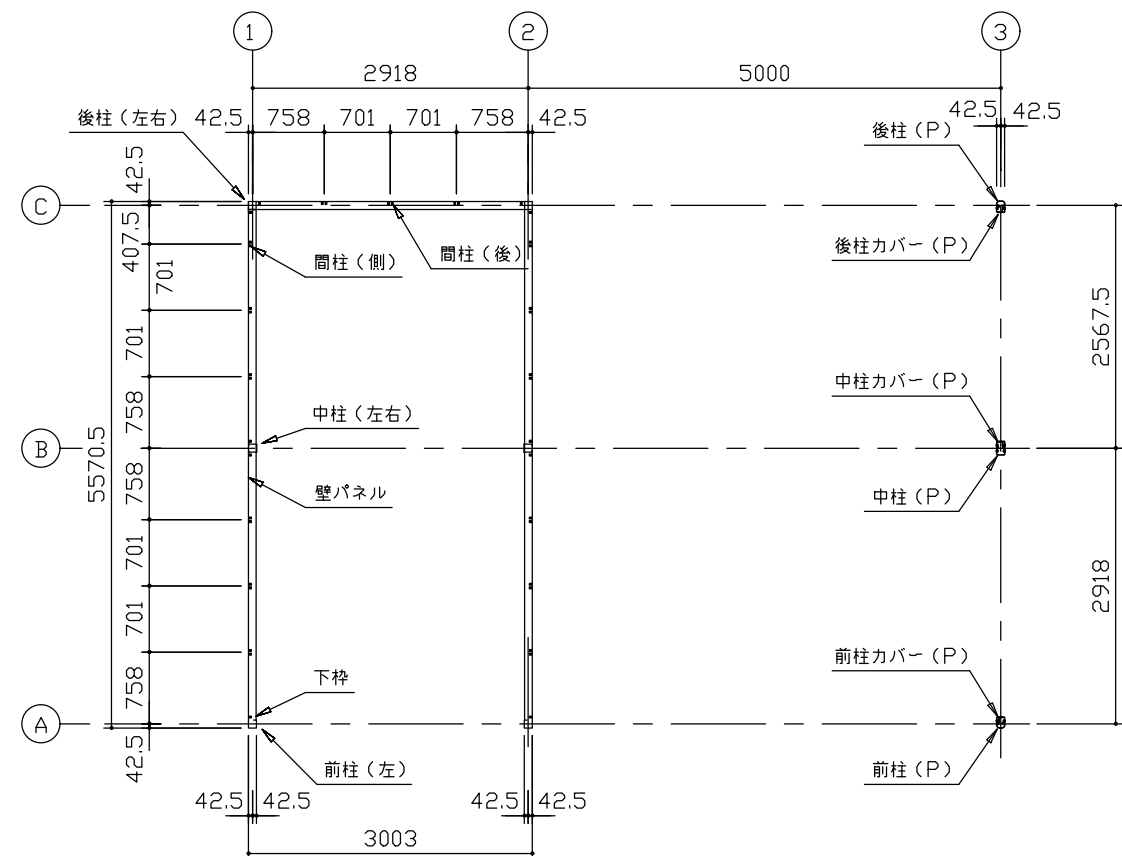
平面図 (S=1/80)
