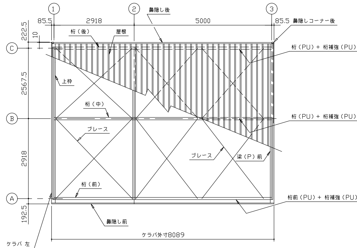
小屋伏図 (S=1/80)
