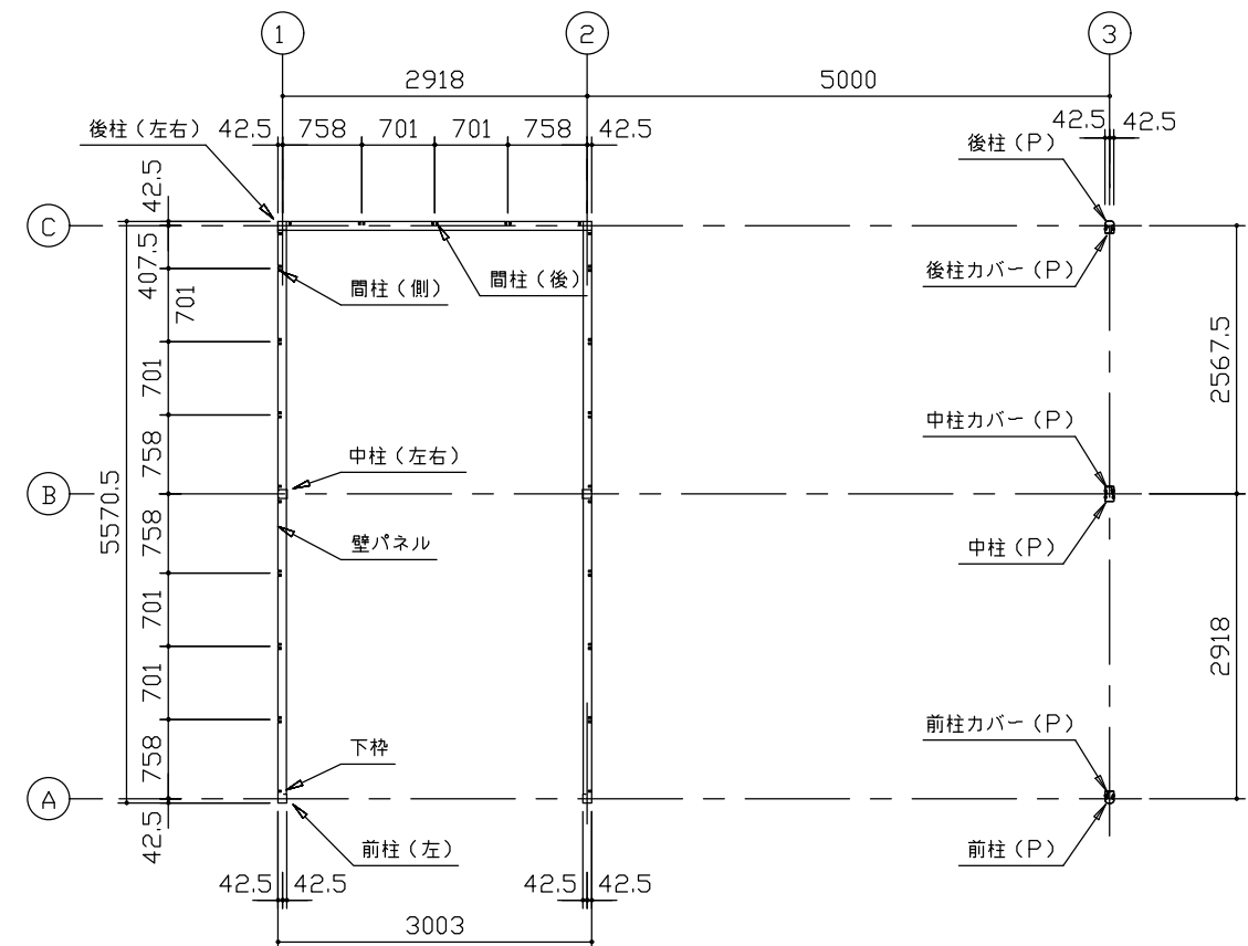
平面図 (S=1/80)
