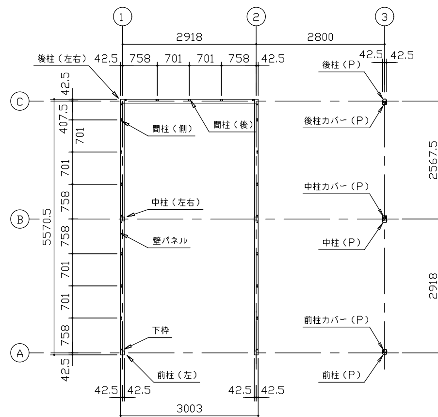
平面図 (S=1/80)
