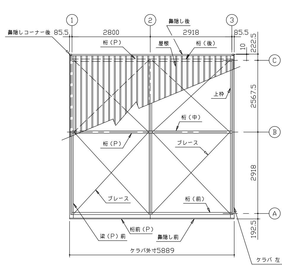
小屋伏図 (S=1/80)
