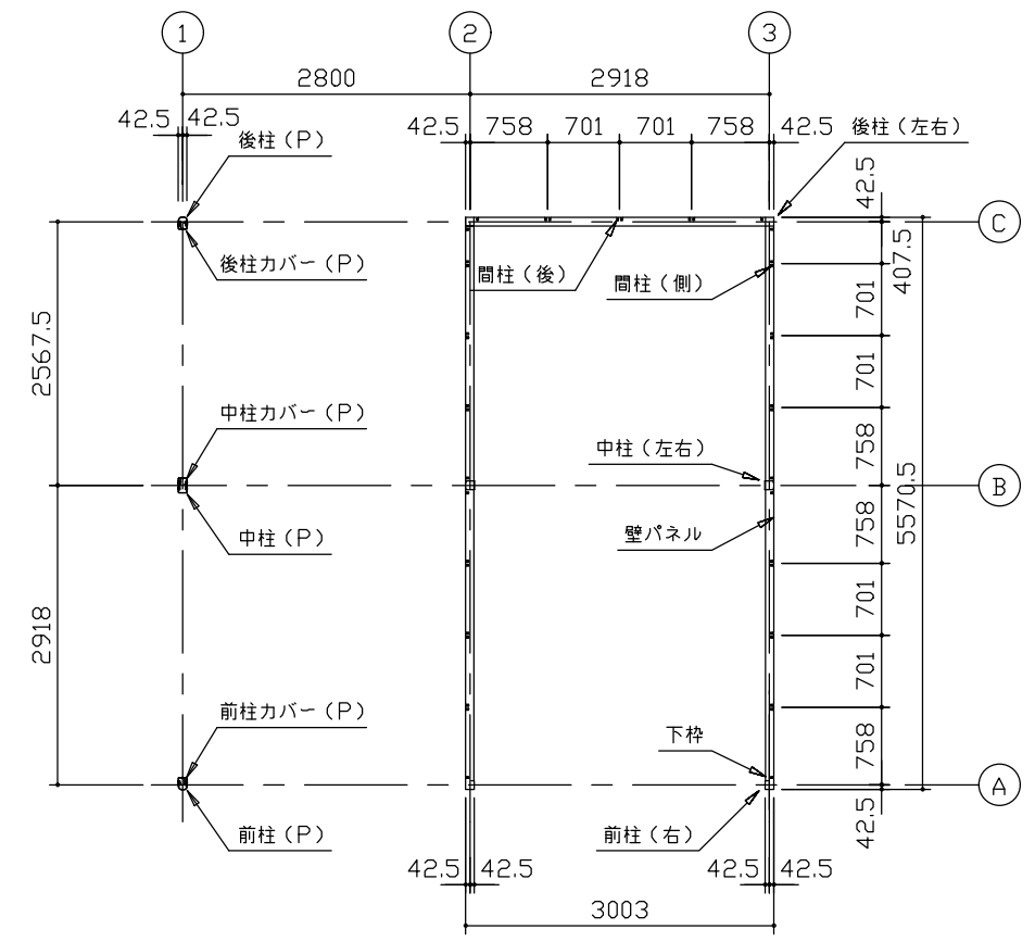
平面図 (S=1/80)
