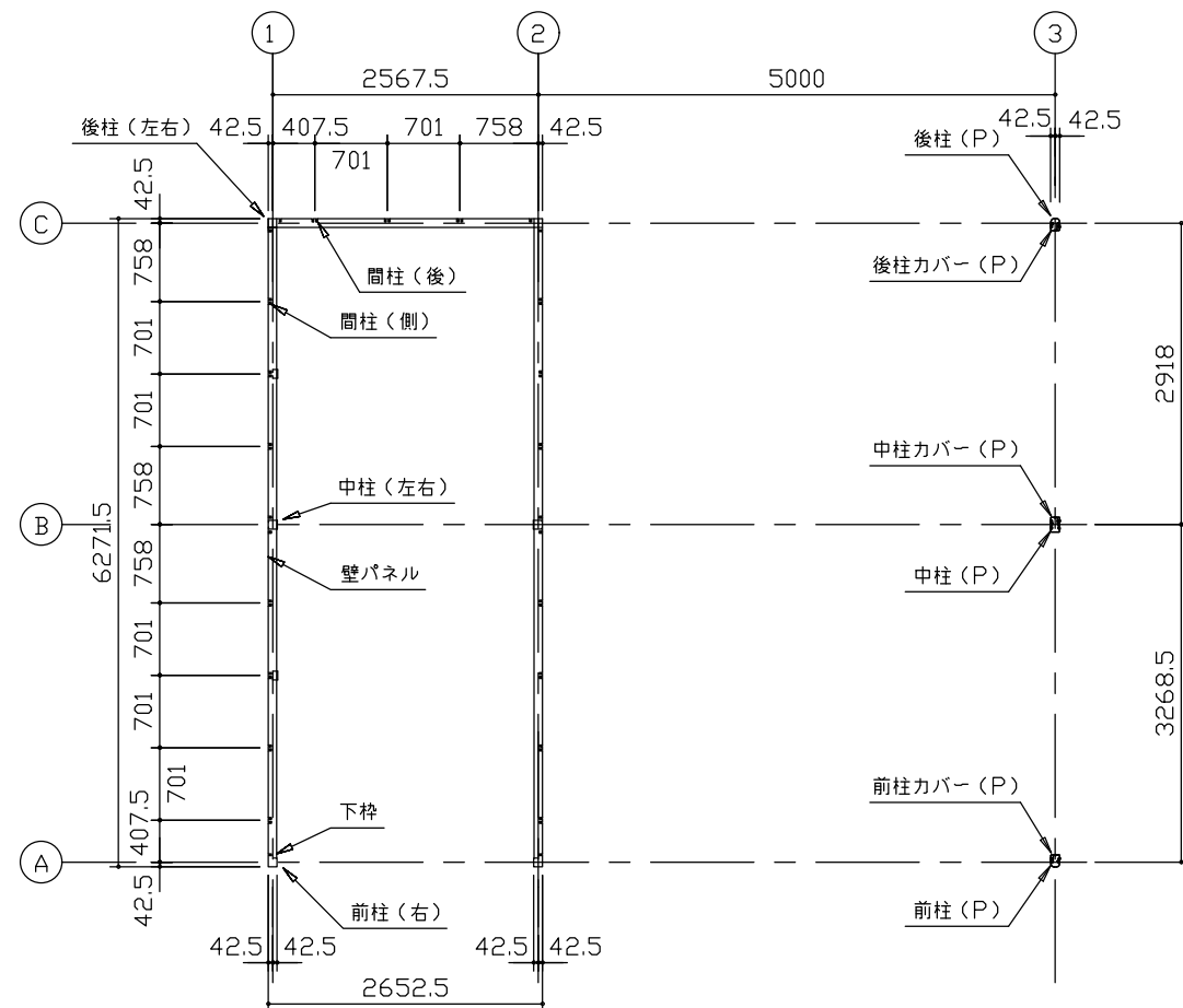
平面図 (S=1/80)
