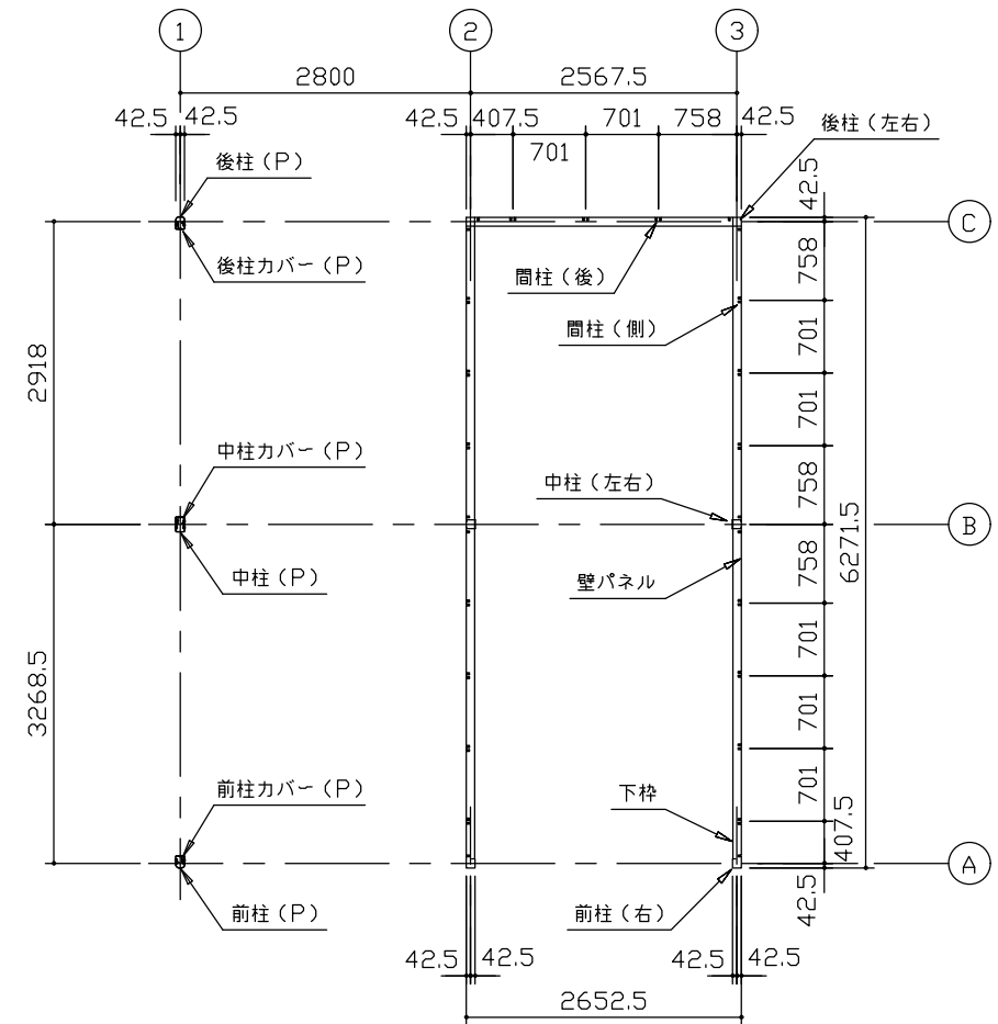
平面図 (S=1/80)
