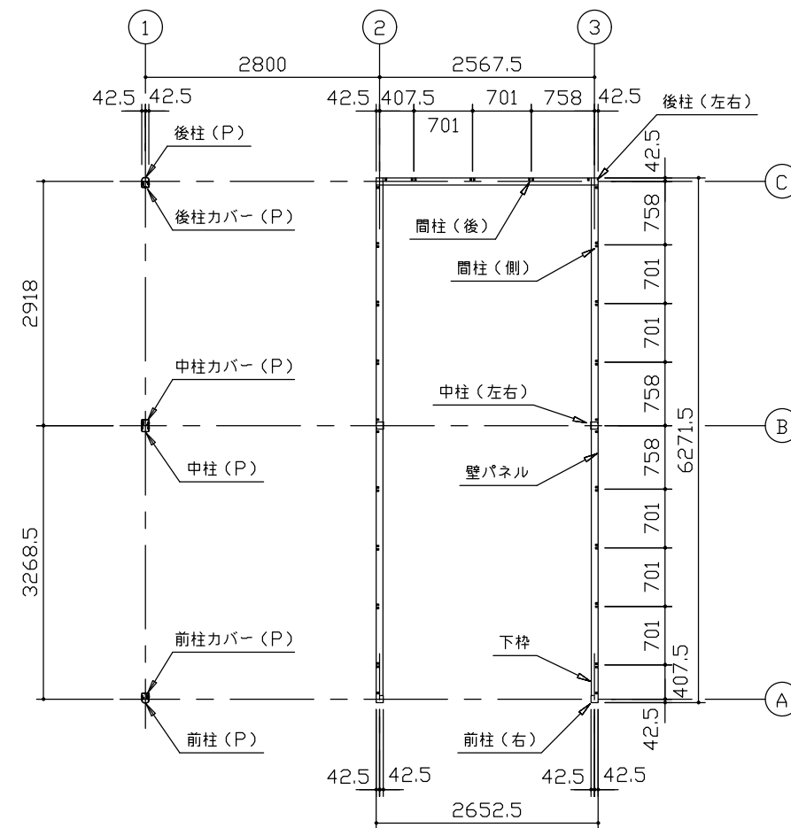
平面図 (S=1/80)
