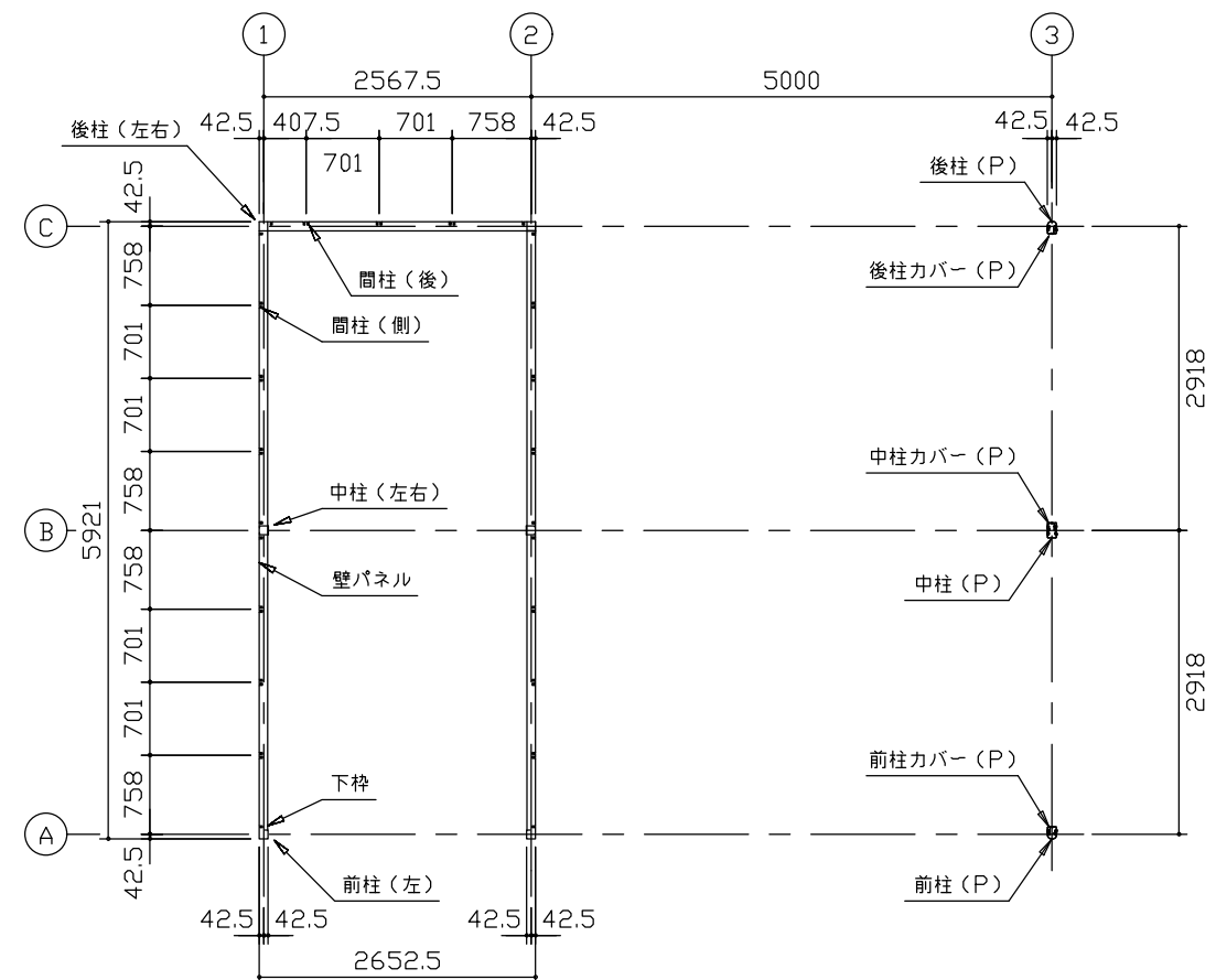
平面図 (S=1/80)
