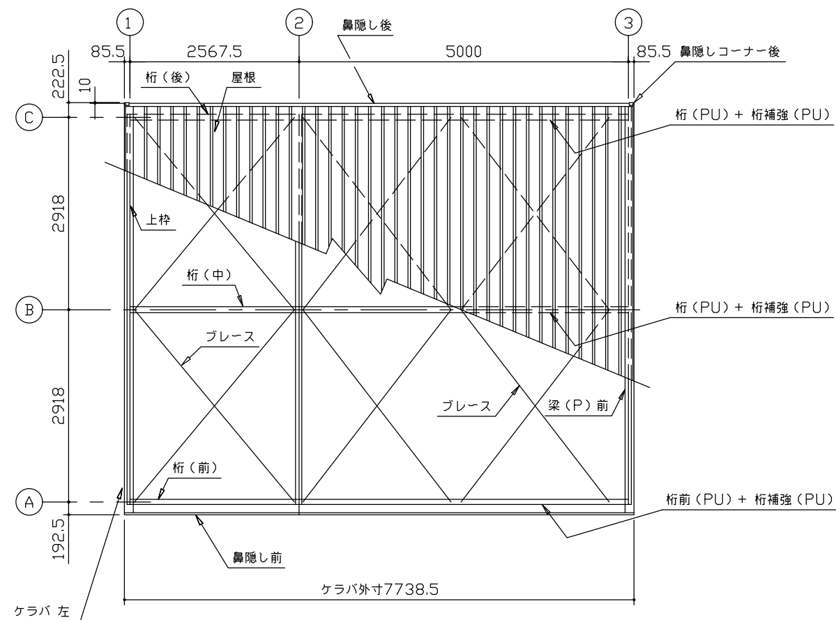
小屋伏図 (S=1/80)
