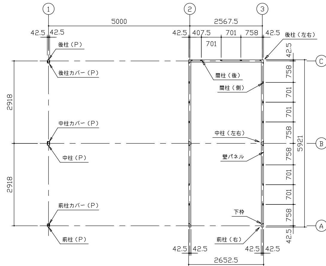
平面図 (S=1/80)
