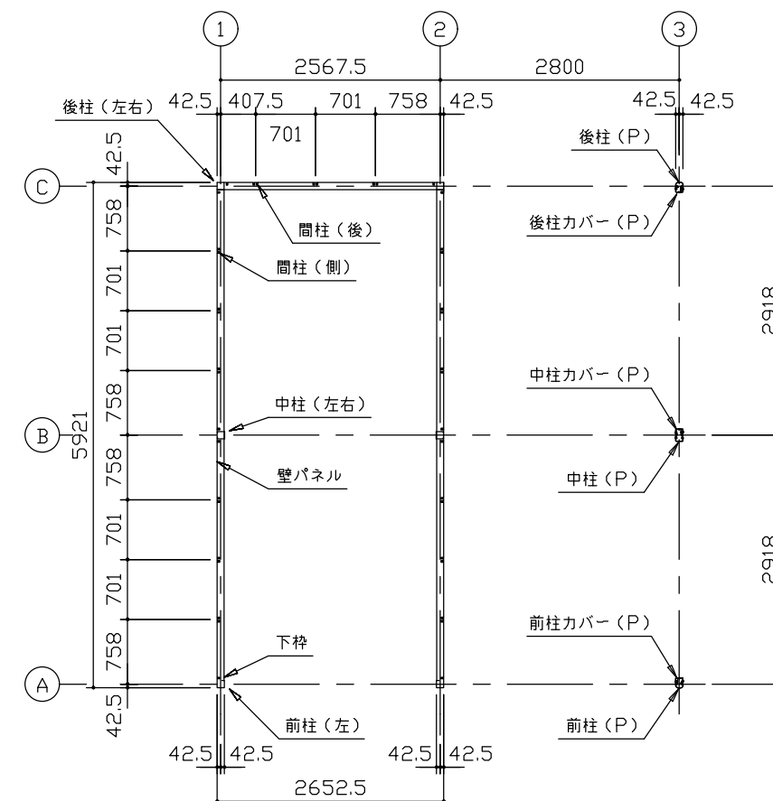
平面図 (S=1/80)
