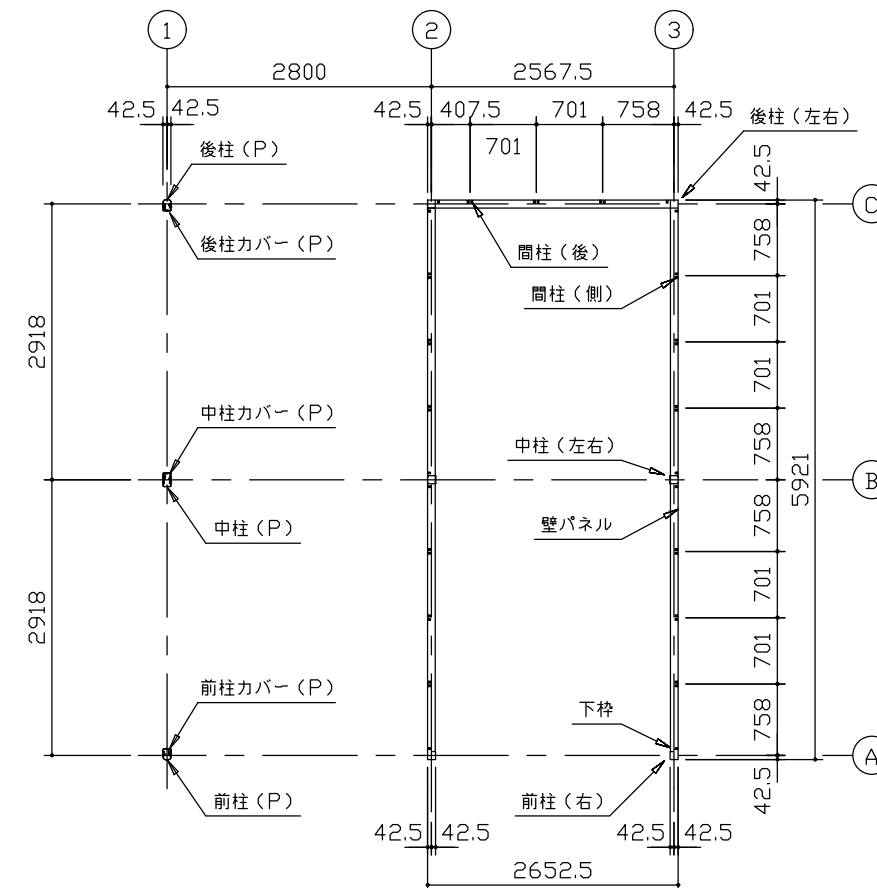
平面図 (S=1/80)
