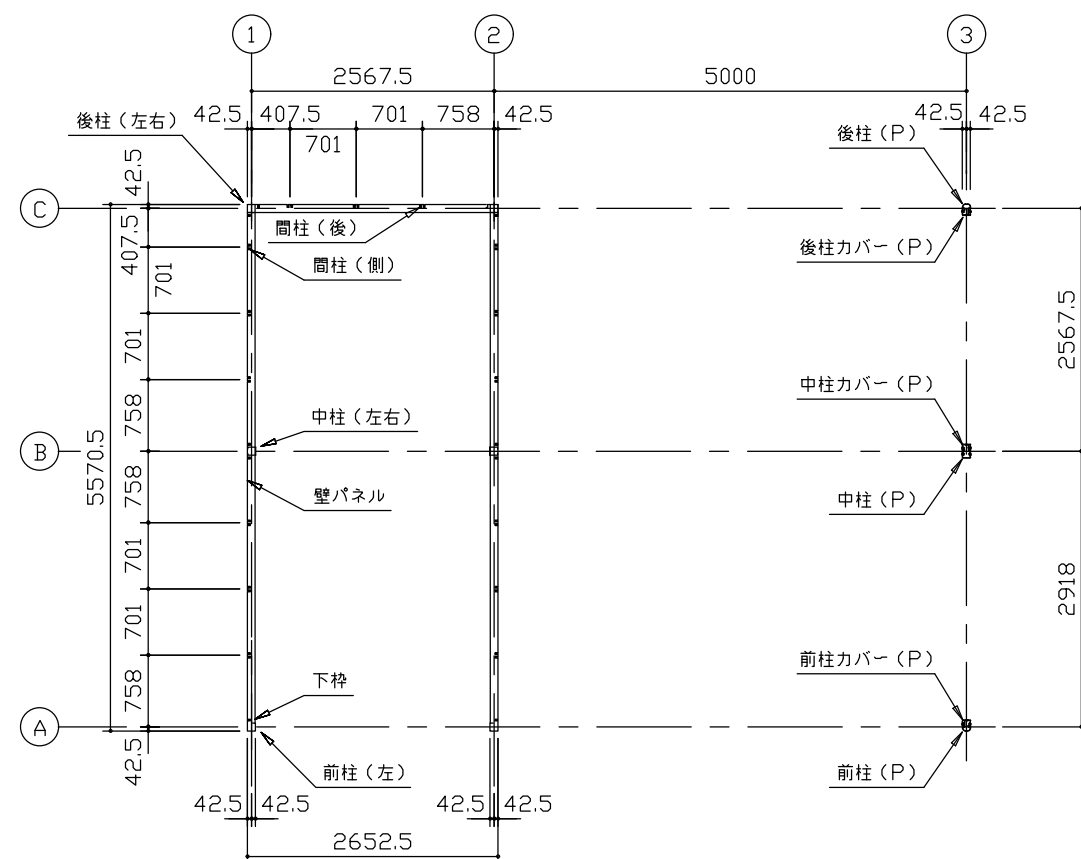
平面図 (S=1/80)
