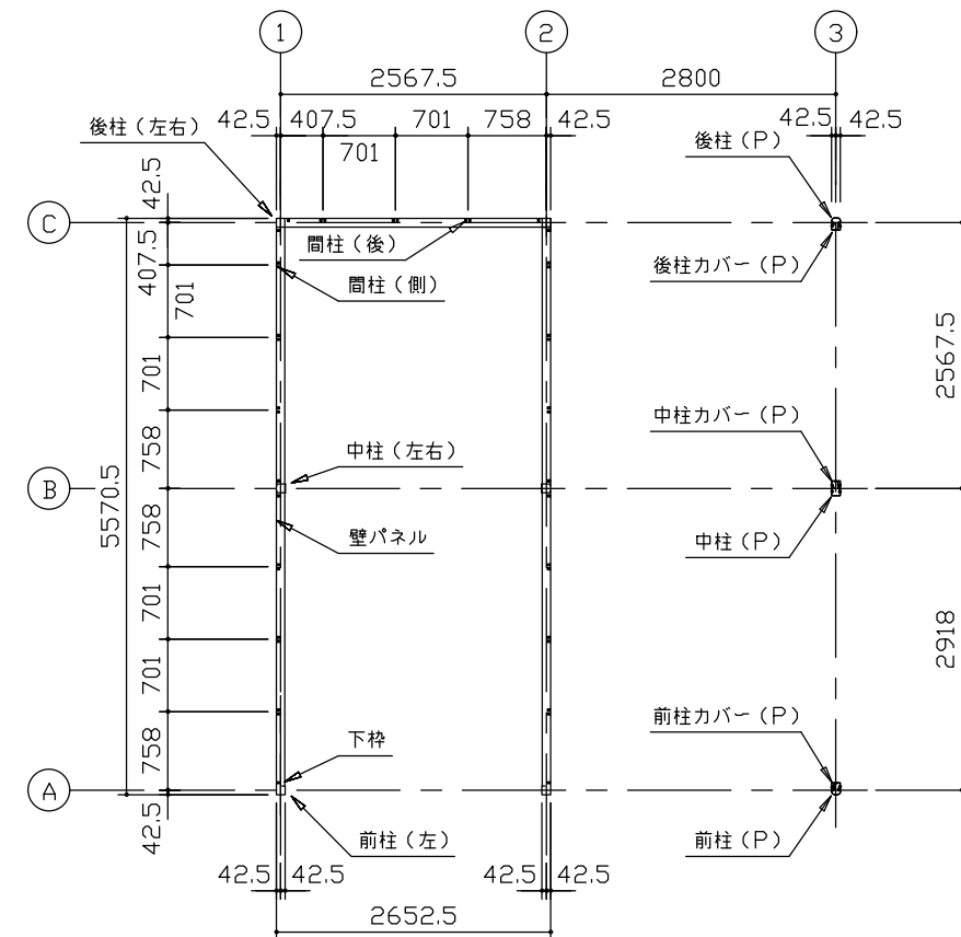
平面図 (S=1/80)
