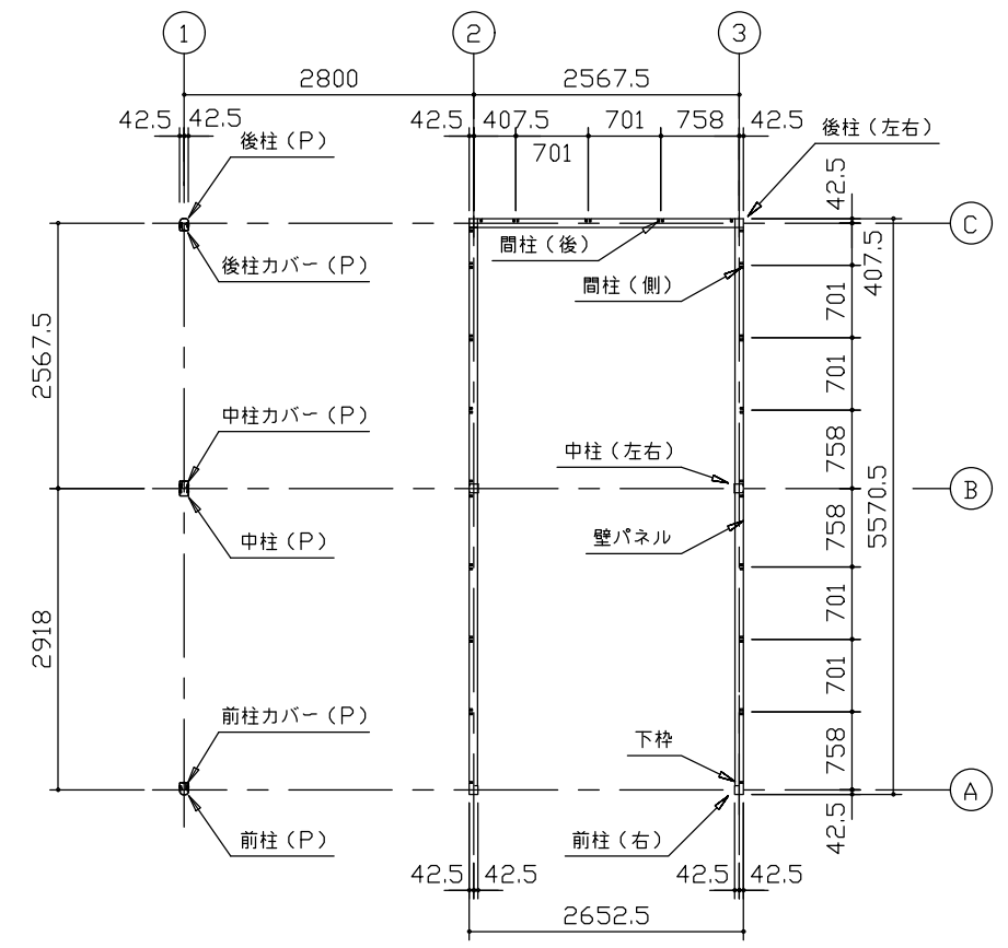
平面図 (S=1/80)
