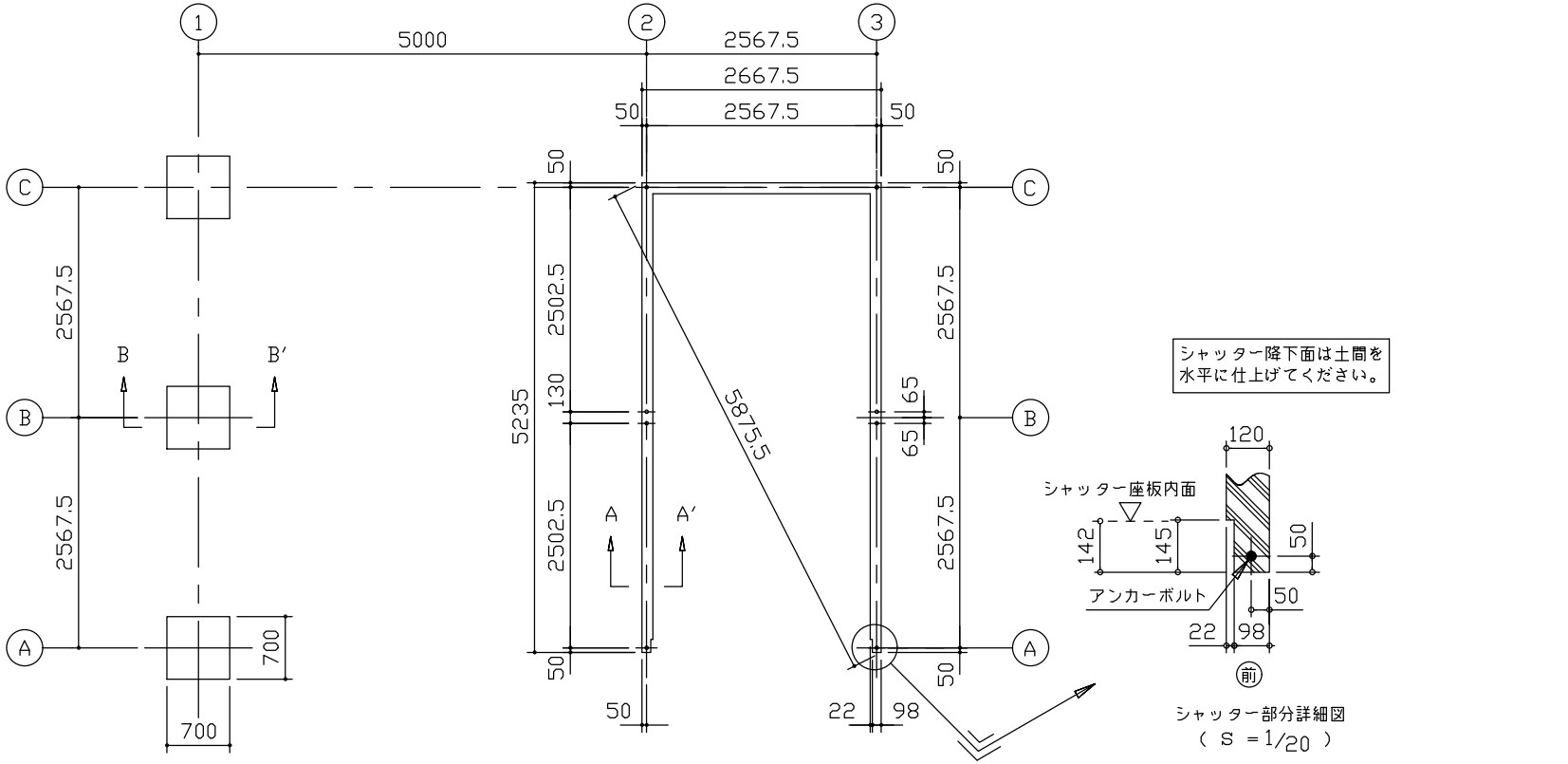
布基礎伏図 (S=1/80)
