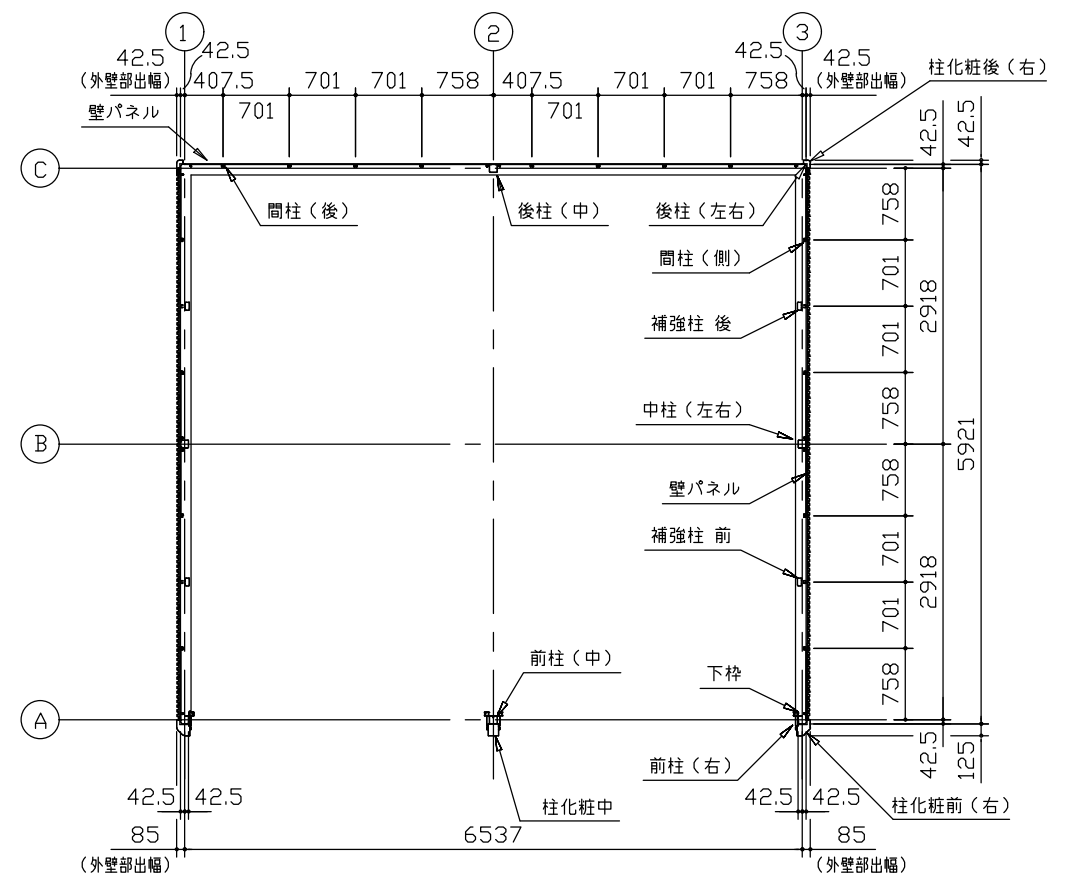
平面図 (S=1/80)
