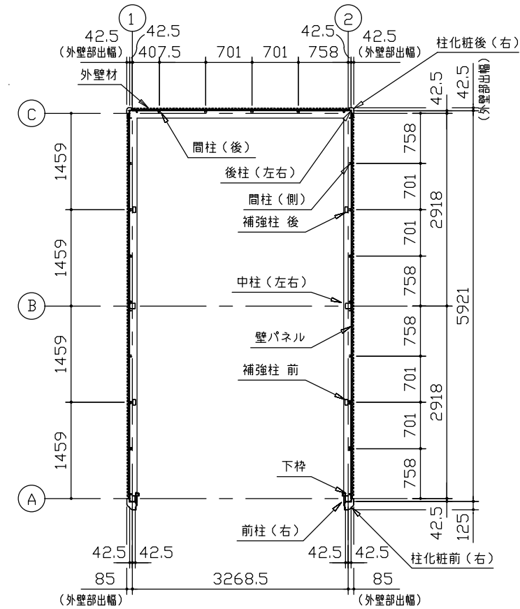
平面図 (S=1/80)
