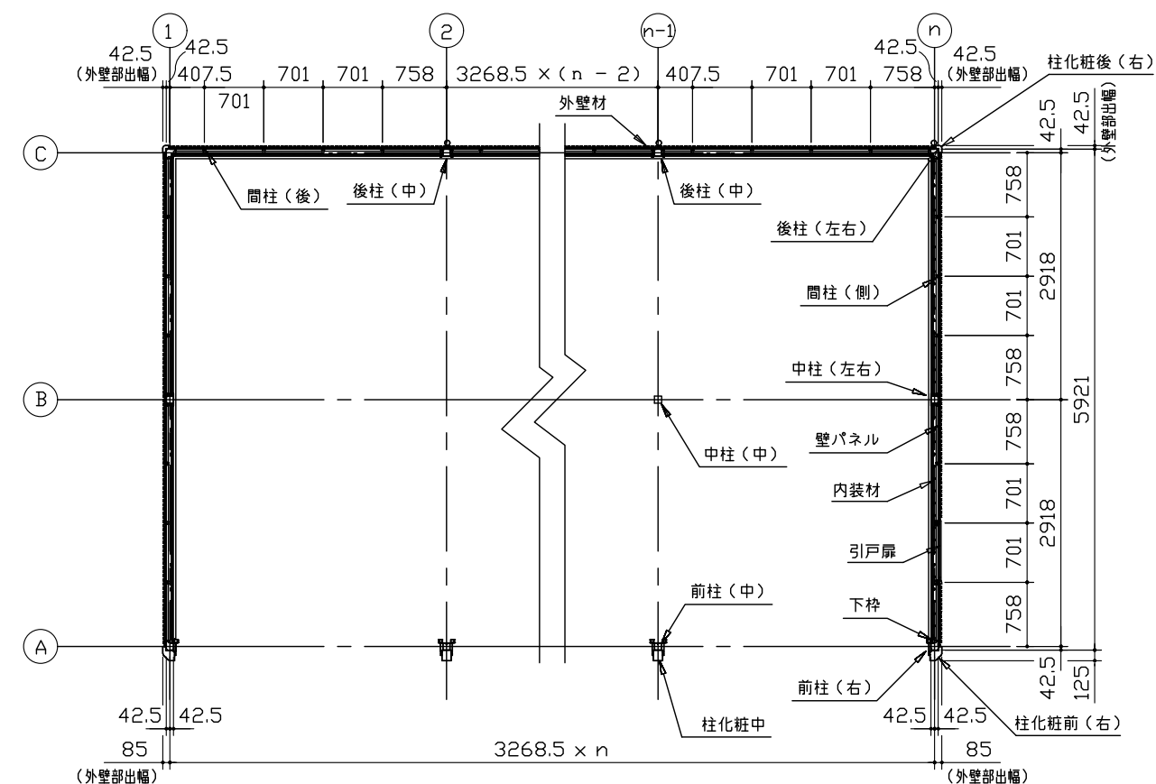
平面図 (S=1/80)
