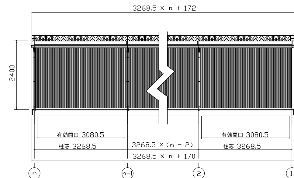
後面立面図 (S=1/80)
