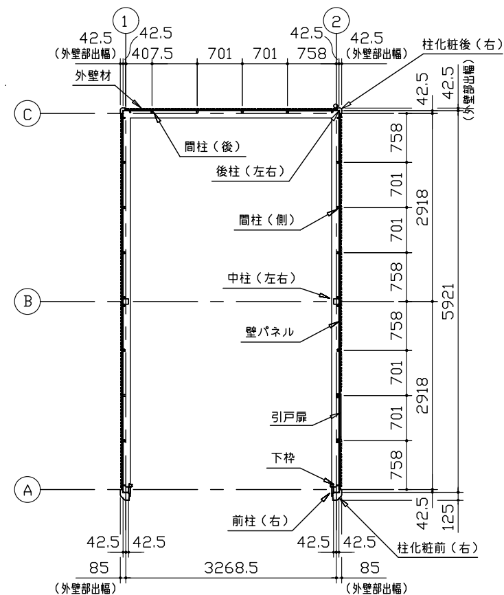
平面図 (S=1/80)
