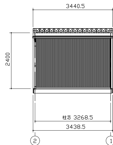
後面立面図 (S=1/80)
