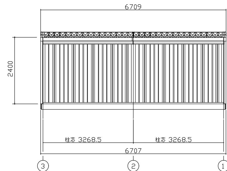
後面立面図 (S=1/80)
