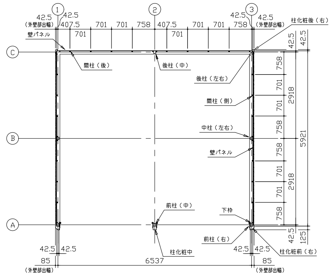
平面図 (S=1/80)
