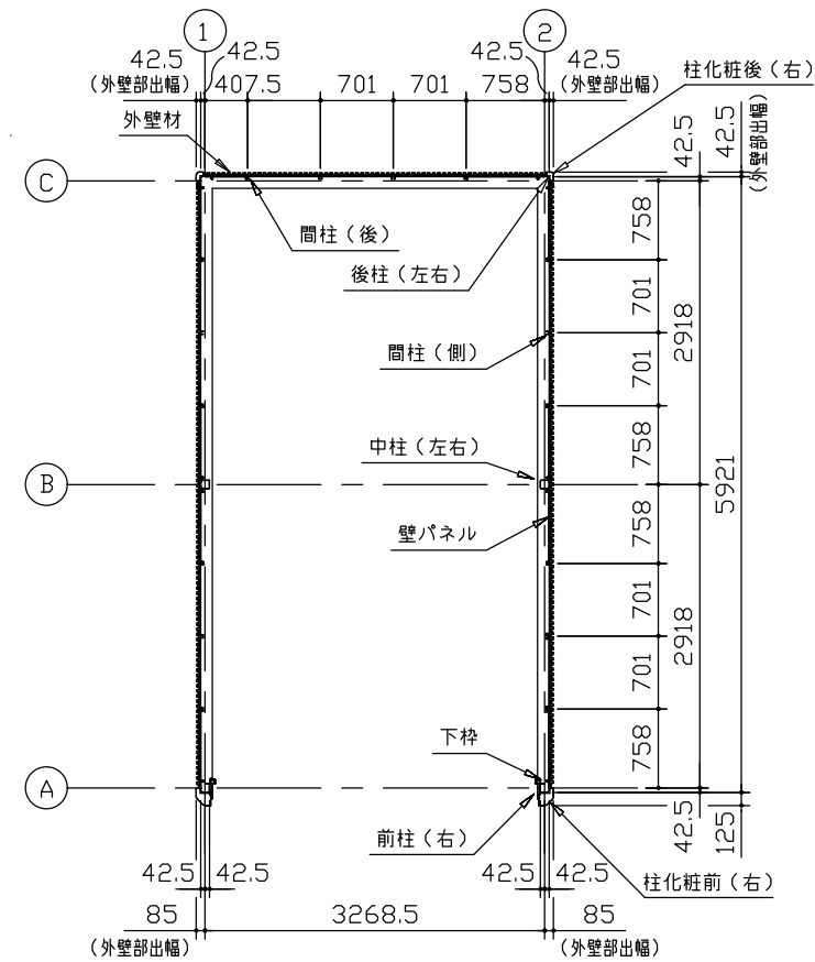
平面図 (S=1/80)
