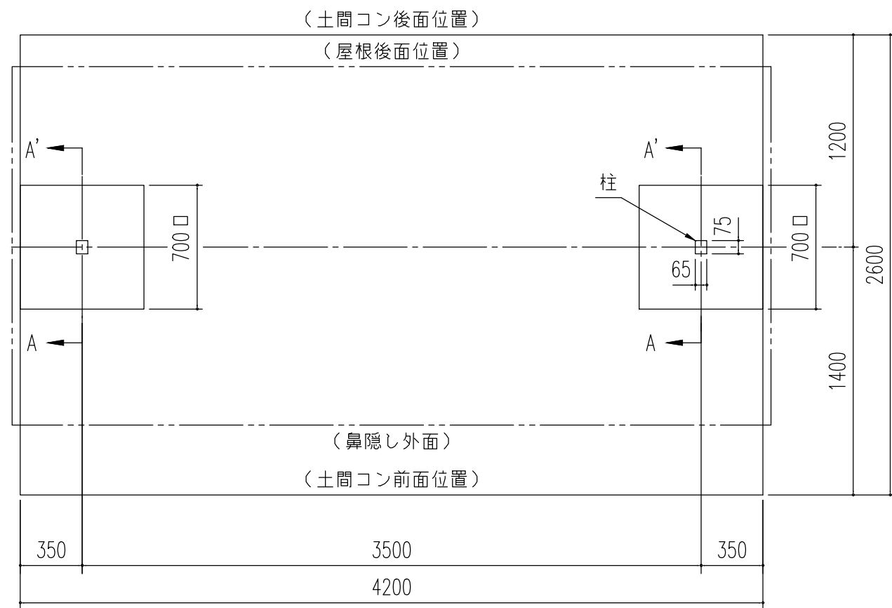
基礎伏図 (S=1/30)
