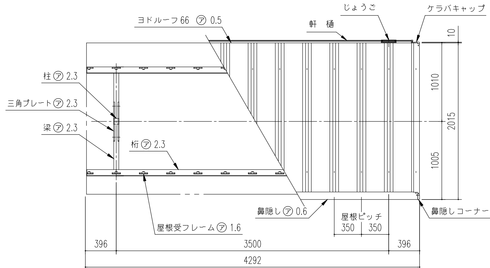
小屋伏図 (S=1/30)
