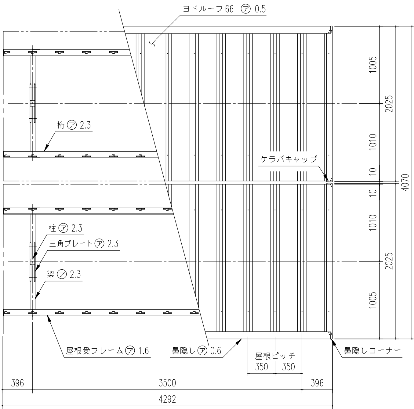
小屋伏図 (S= 1/30)
