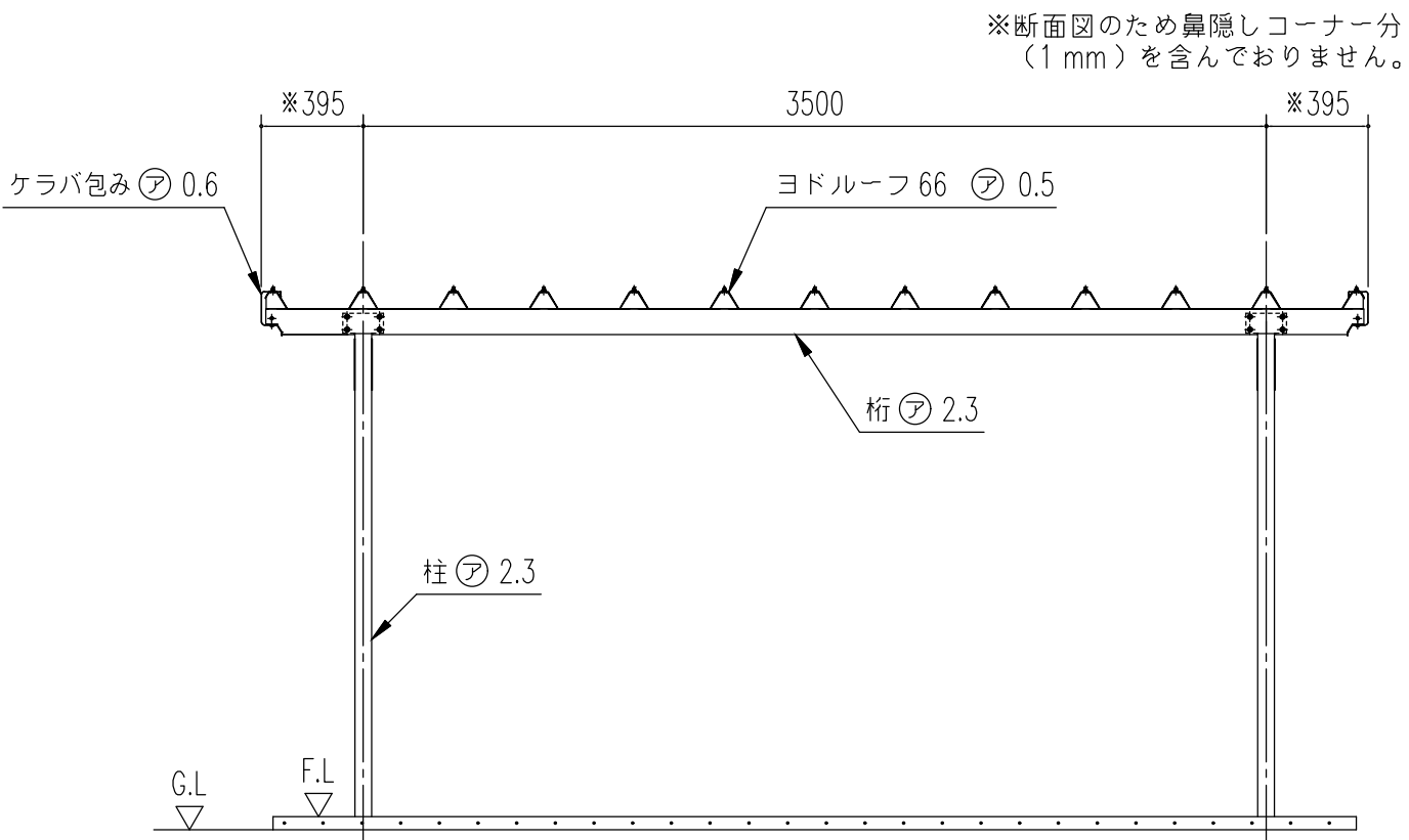
正面断面図 (S= 1/30)
