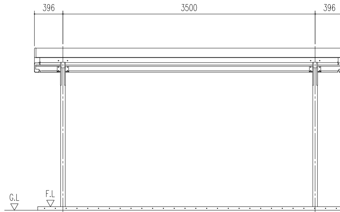
正面立面図 (S= 1/30)
