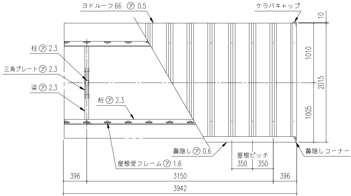
小 屋 伏 図 (S= 1/30)
