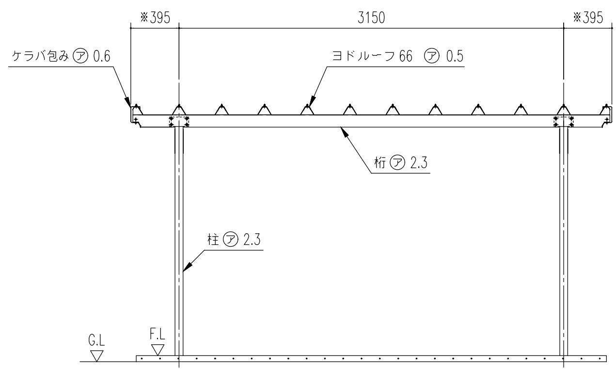
正面断面図 (S= 1/30)
