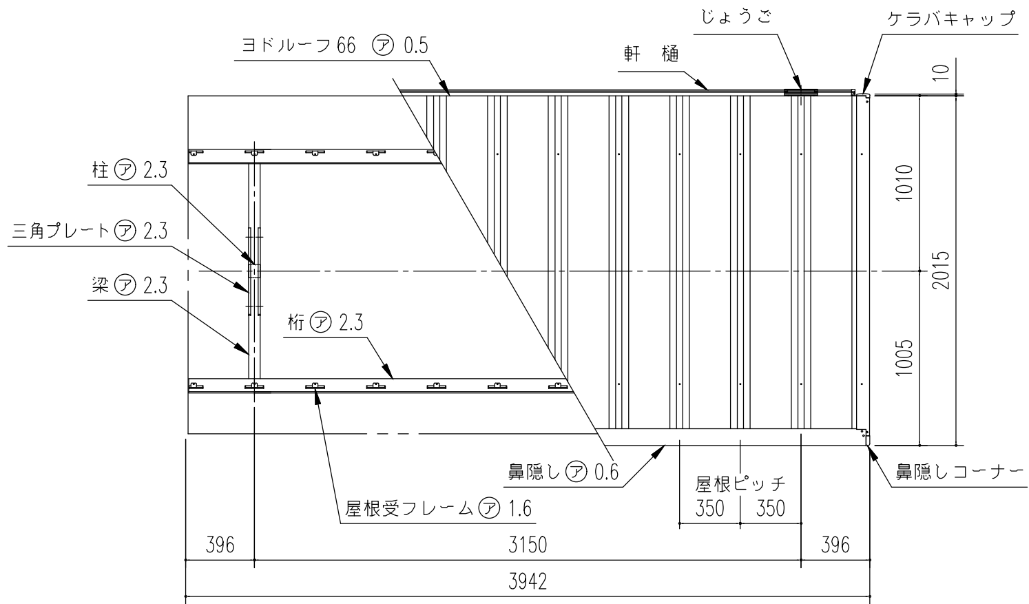
小屋伏図 (S= 1/30)
