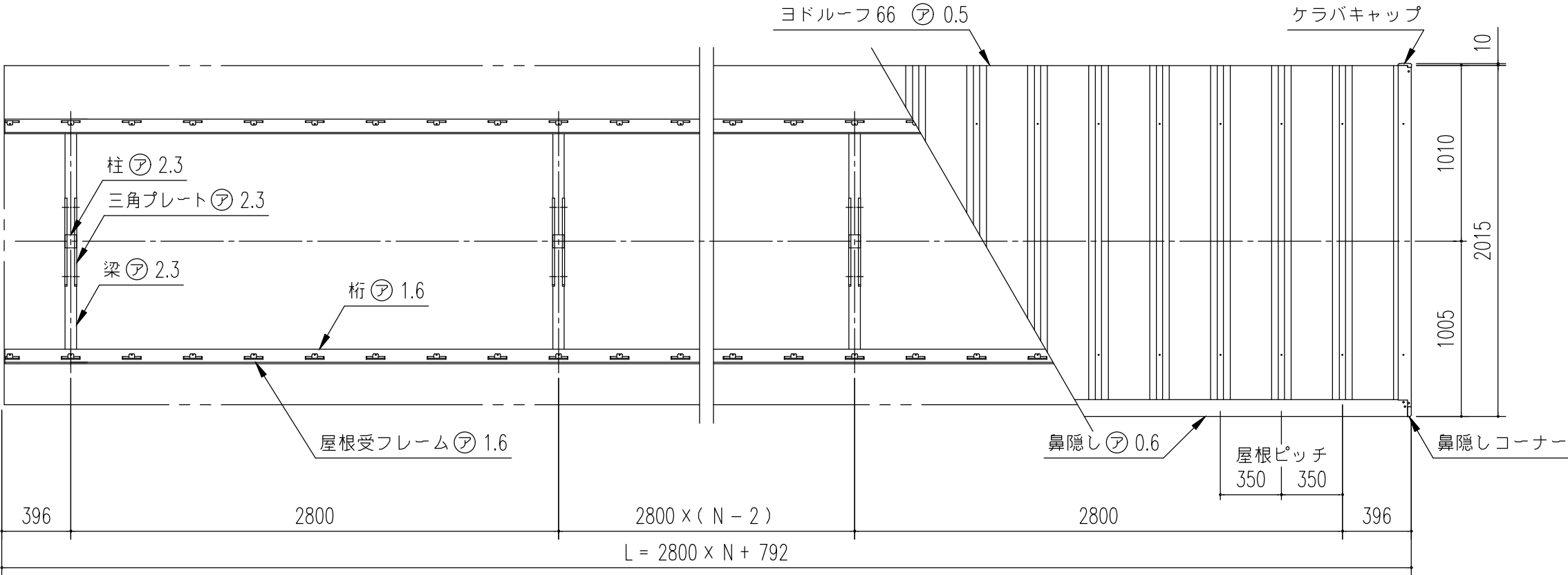
小屋伏図 (S=1/30)
