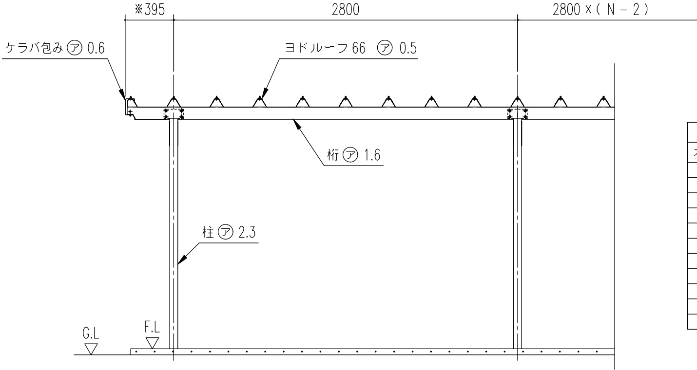
正面断面図 (S=1/30) ( N : スパン数 )
