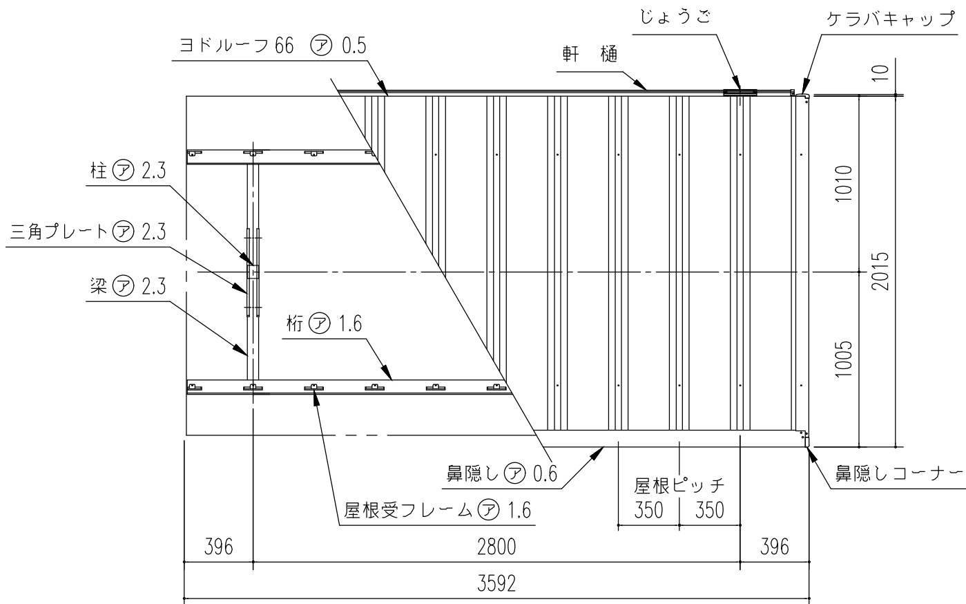
小 屋 伏 図 (S= 1/30)
