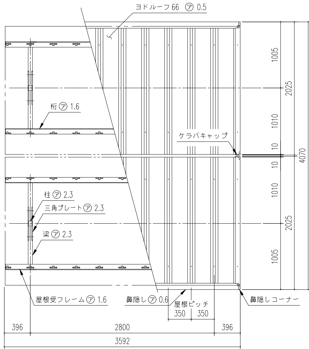
小屋伏図 (S= 1/30)
