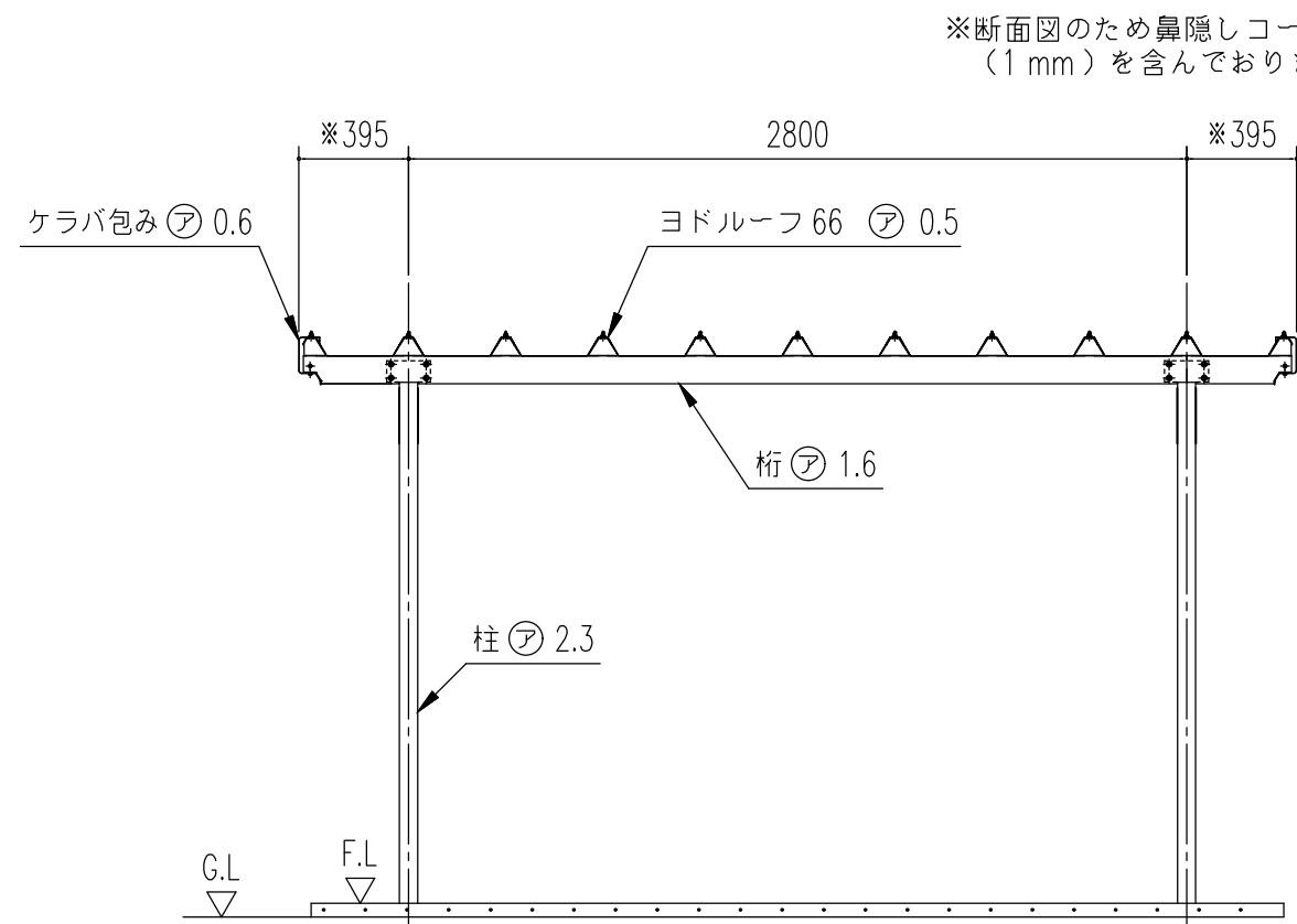
正面断面図 (S= 1/30)
